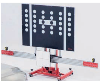
ADAS Compatible
